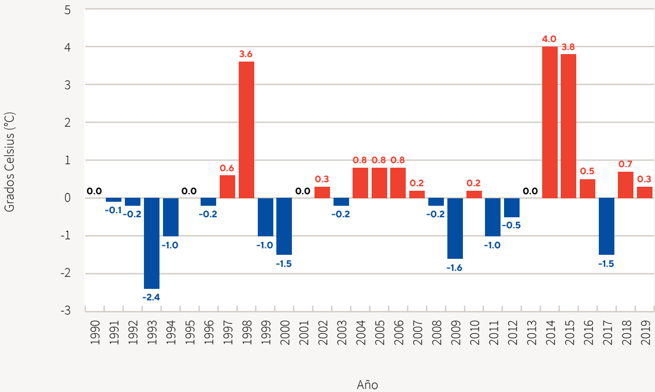
Gráfico 15. Temperatura mínima extrema anual (arriba) y temperatura mínima extrema anual promedio por décadas (abajo) en Coronel Oviedo, Caaguazú (Barra roja T > 0^{\circ}\text{C} y barra azul T < 0^{\circ}\text{C} ). Período 1990-2019.
