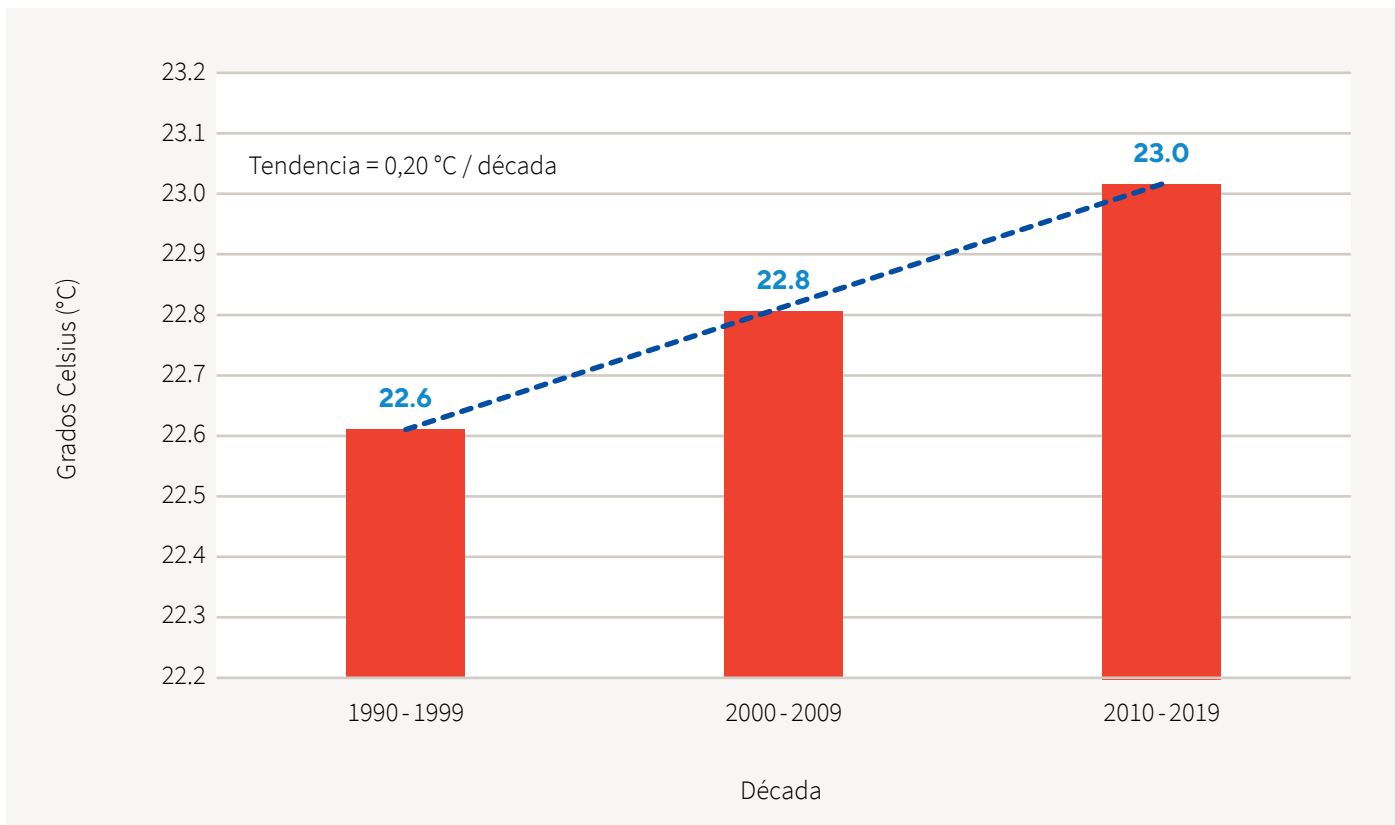
Gráfico 7. Temperatura media decadal en Coronel Oviedo, Caaguazú. Período 1990-2019.
